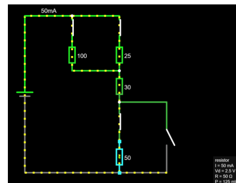
Falstad Circuit
