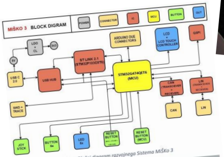
Slika 1: Bločni diagram razvojnega Sistema Miška 3
