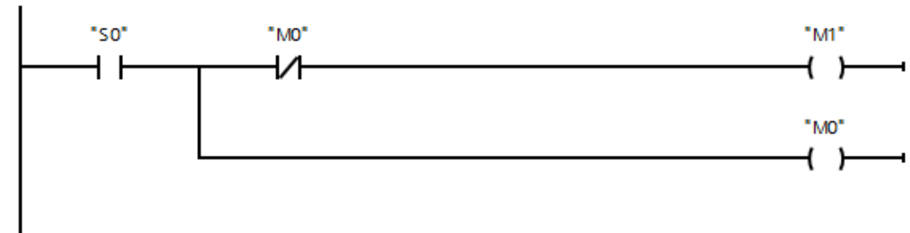
Network 1: Detekcija pozitivne fronte na S0
